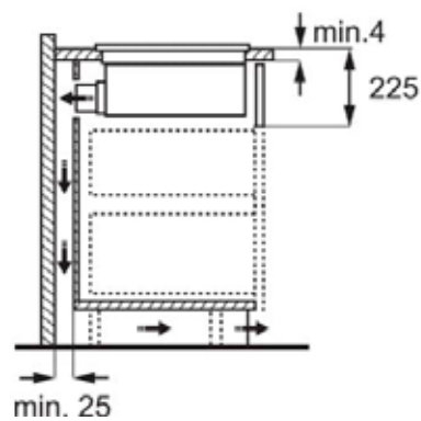
Schéma d'encastrement
